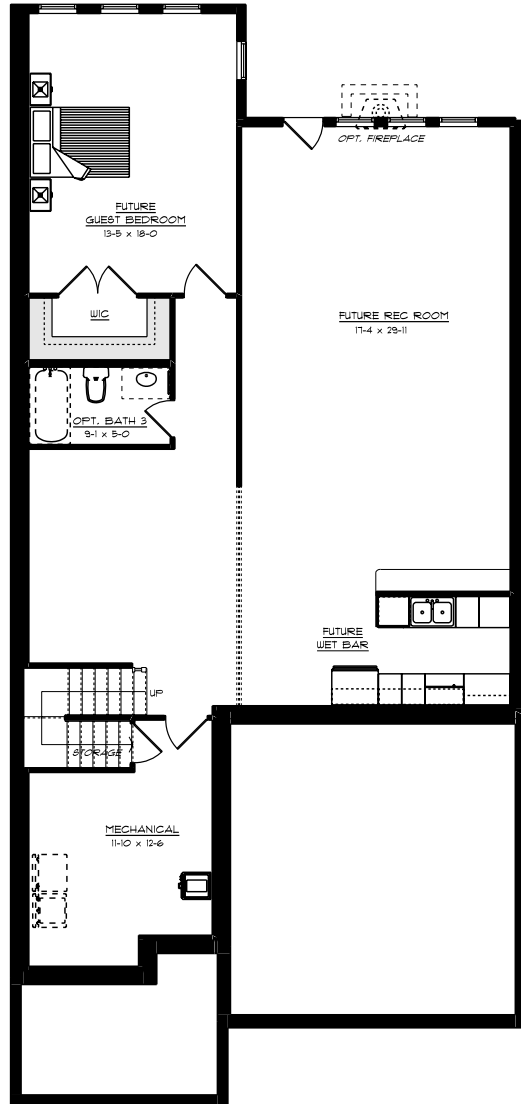
OPTIONAL BASEMENT
